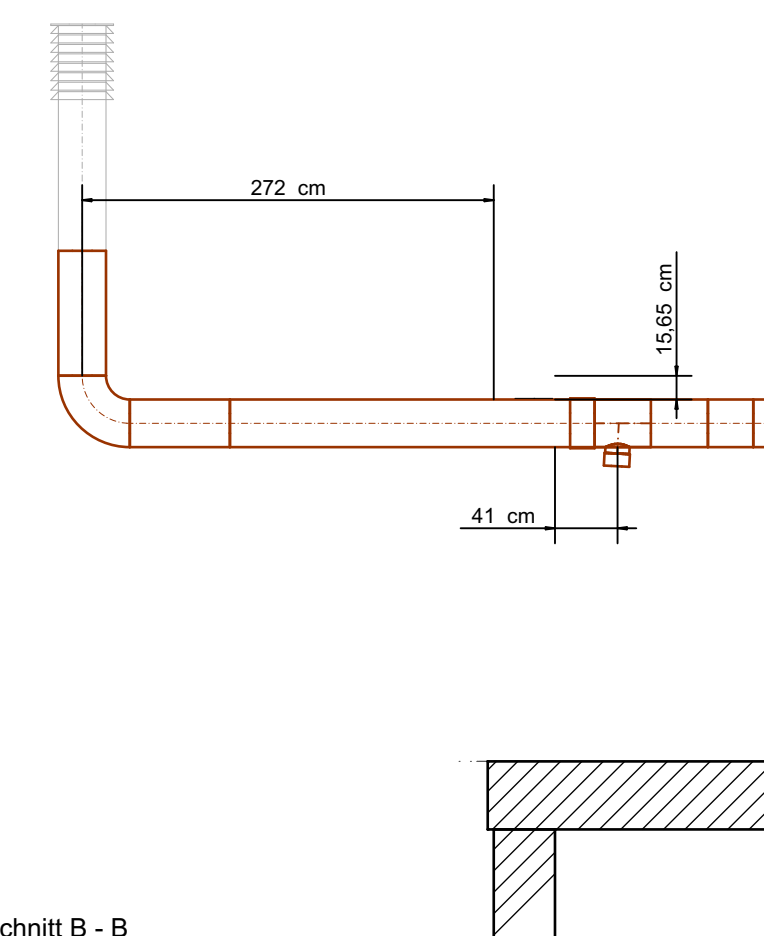
Schnitt B - B
