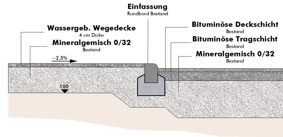
Gebundene Decke - Asphalt
