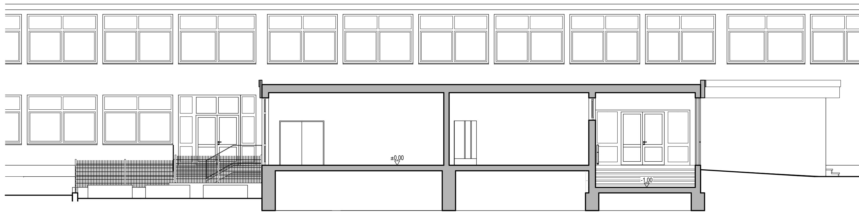
SCHNITT C-C
