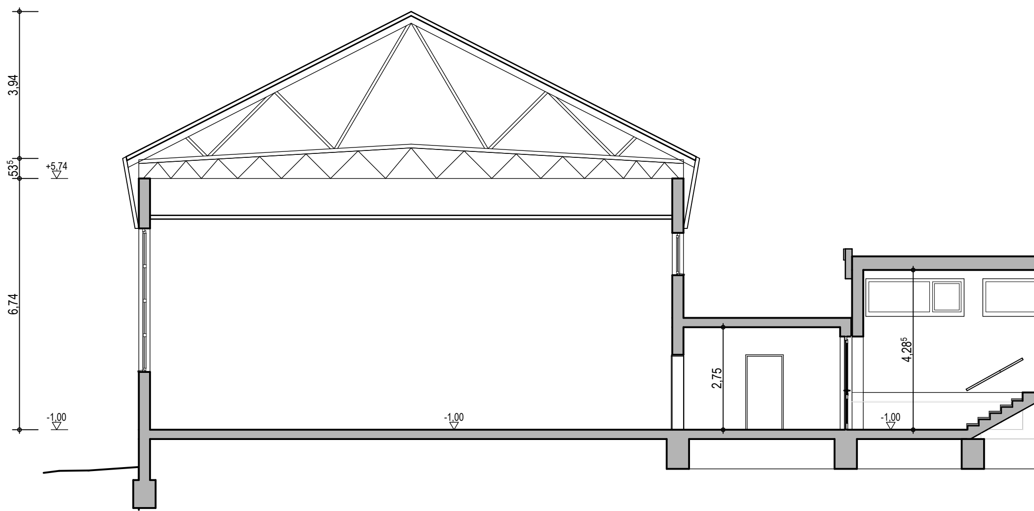
SCHNITT D-D
